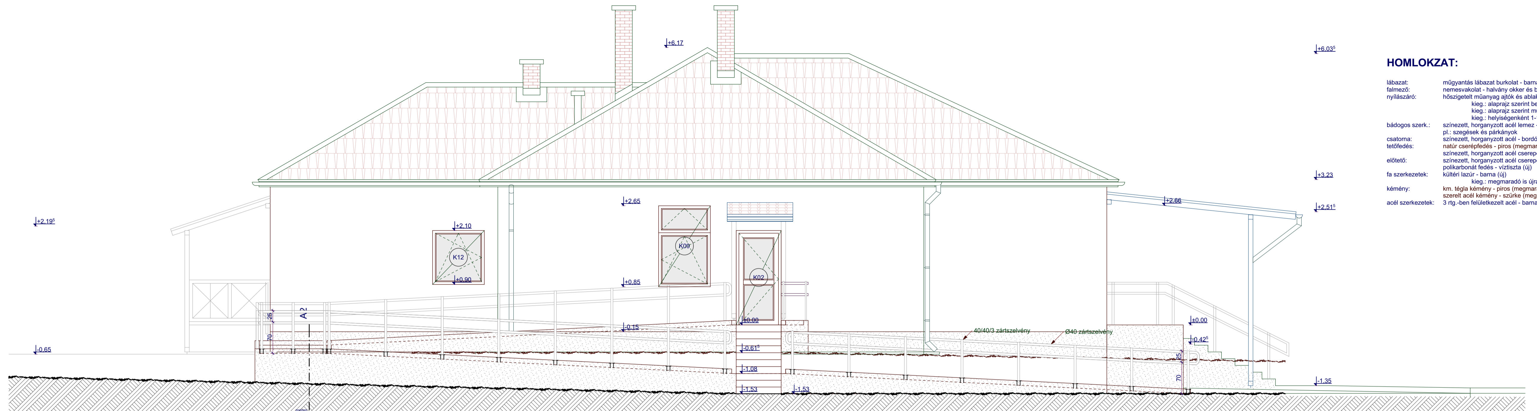
Keleti homlokzat
