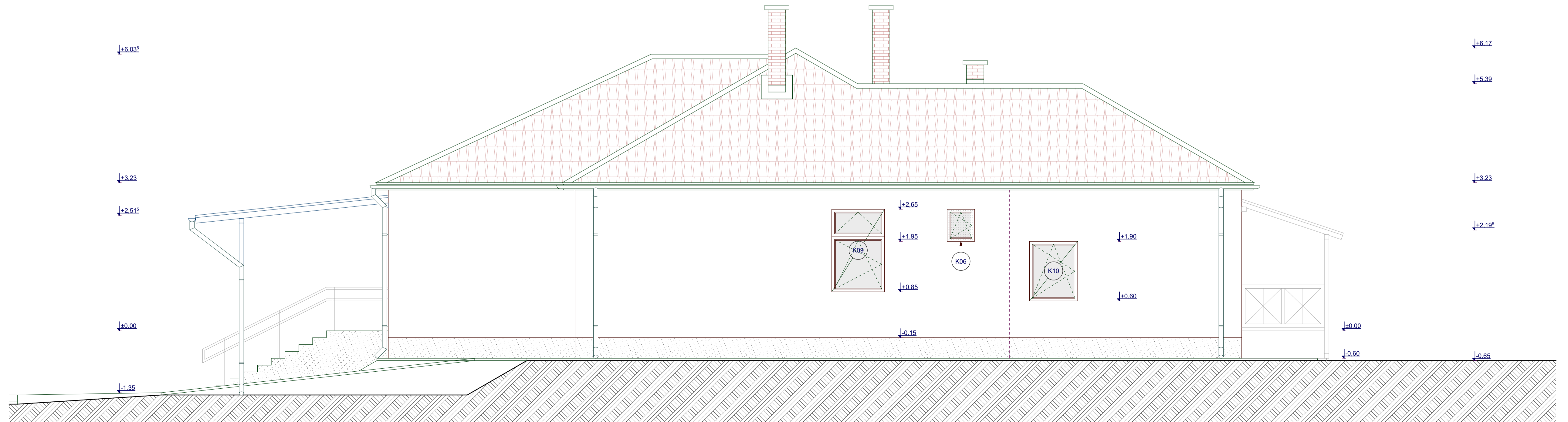
Nyugati homlokzat
