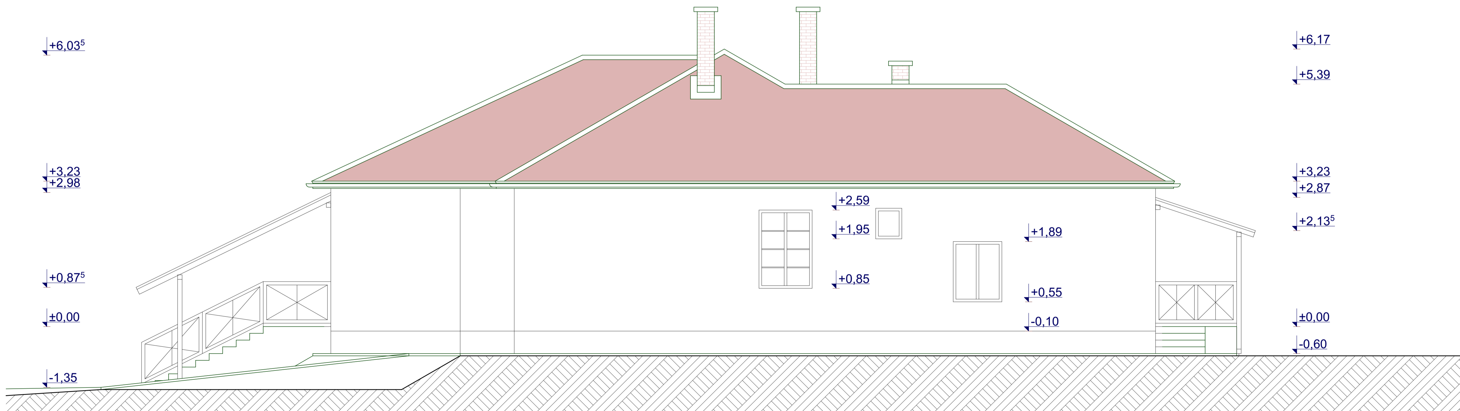
Nyugati homlokzat
